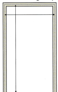
Door Nominal Door Width + 1 1/4" Jamb Height + 1"
